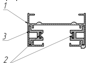
Конструкция шинопровода однофазного Geniled.
