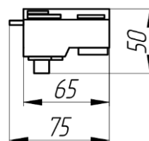
Адаптер для однофазного шинопровода Geniled
