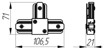
Соединитель T Geniled для однофазного шинопровода
