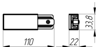
Ввод питания для однофазного шинопровода
