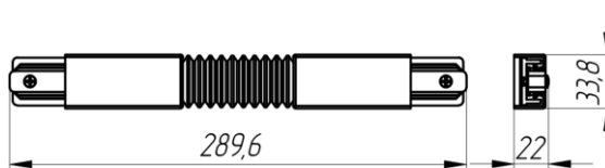
Соединитель гибкий в гофре Geniled для однофазного шинопровода
