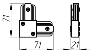
Соединитель L Geniled для однофазного шинопровода
