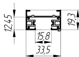
Габаритные размеры шинопровода однофазного Geniled.
