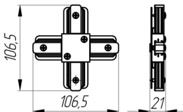
Соединитель X Geniled для однофазного шинопровода
